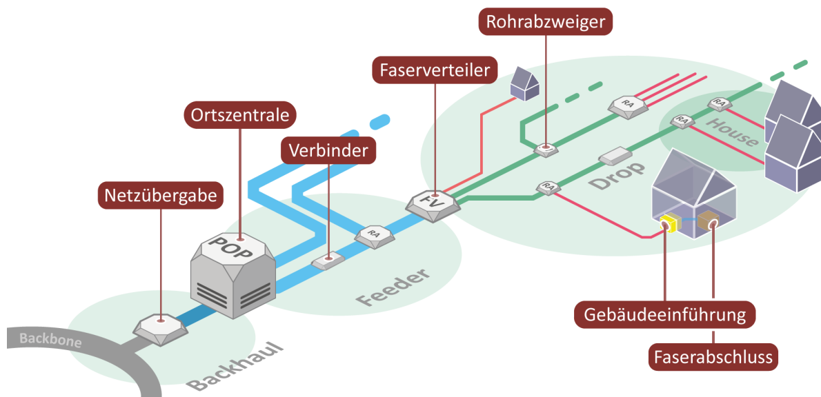
Abb. 2 - FTTH Netzstruktur
