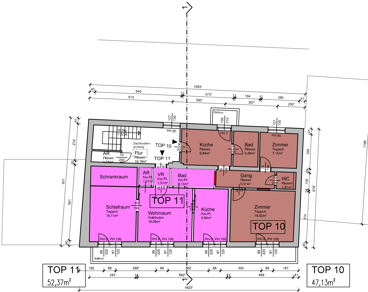
GRUNDRISS 2. OBERGESCHOSS
